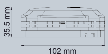
尺寸圖
