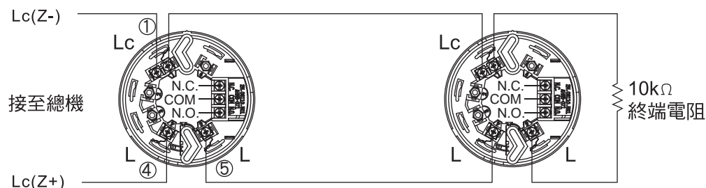
Type 3 四線式 附接點輸出 最大負載規格： DC 30V / 0.8A AC 125V / 0.4A
