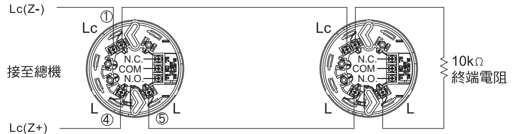
Type 3 四線式 附接點輸出 最大負載規格： DC 30V / 0.8A AC 125V / 0.4A
